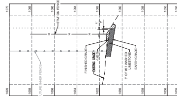
SECTION F VERTICAL SCALE: 1" = 2' HORIZONTAL SCALE: 1" = 20'
