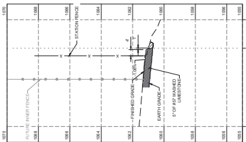
SECTION E VERTICAL SCALE: 1" = 2' HORIZONTAL SCALE: 1" = 20'
