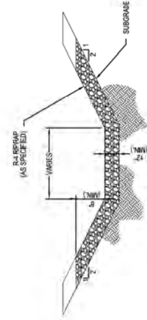
RIPRAPPED CHANNEL SCALE: N.E.S.
